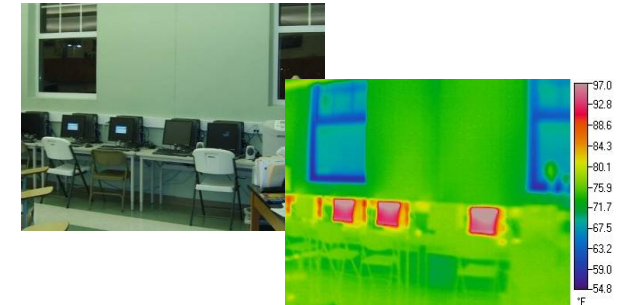
Thermographie einer THERMOMASS® Wand
