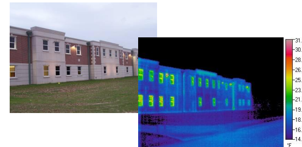
Thermographie einer herkömmlichen Wand
