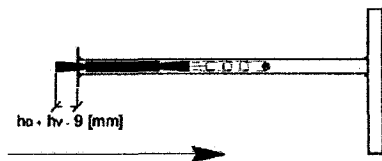
3. TMDW Anker in die TMDW Setzhilfe einführen
