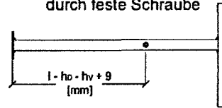
2. TMDW Setzhilfe mit Tiefenbestimmung durch feste Schraube
