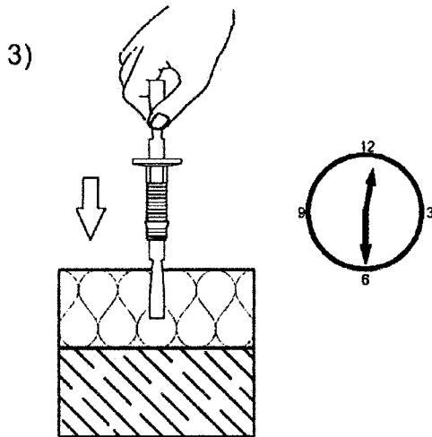
3) TMDW-Anker mit Manschette bis zum Anschlag einsetzen
