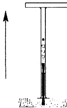
7. TMDW Setzhilfe hochziehen ohne den TMDW Anker wieder hinauszuziehen
