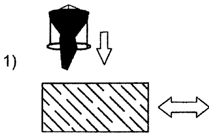
1) Beton der Vorsatzschicht einfüllen und verdichten
